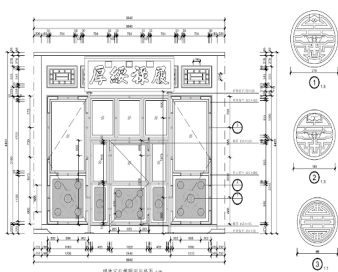
图1 翊坤宫明间外檐装修图
