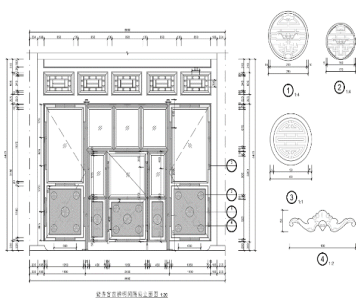
图2 储秀宫明间外檐装修图
