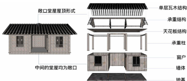
图3 敞口堂屋内部结构示意图（图片来源：作者自绘）
