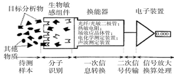
图 2 生物传感器原理
