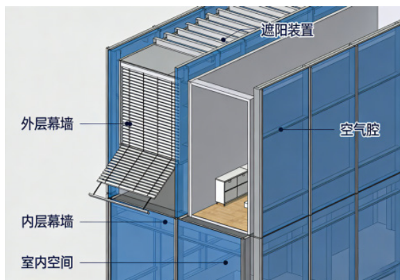
图 1 双层呼吸式幕墙结构示意图
