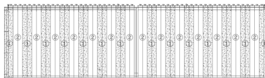
图 5 跳仓法浇筑平面布置示意图
