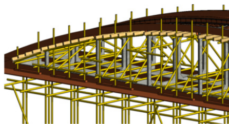
图 2 搭设体系大样图
