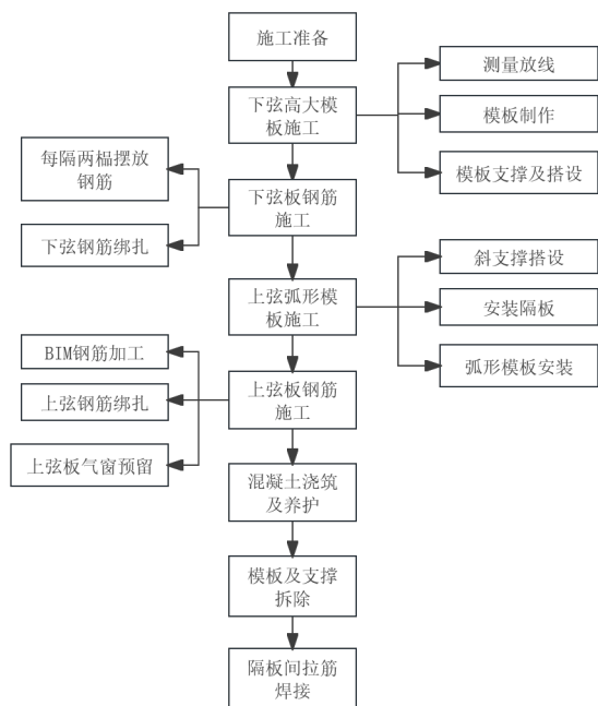
图 1 施工工艺流程图
