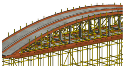
图 7 上下弦屋面板混凝土浇筑完成示意图
