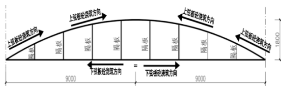
图 6 混凝土浇筑顺序示意图
