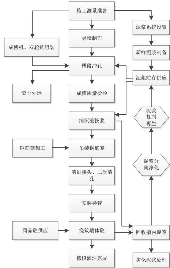
图1 地下连续墙流程图示意图
