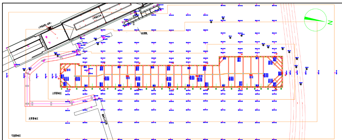
图2 基坑施工监测平面布置图
