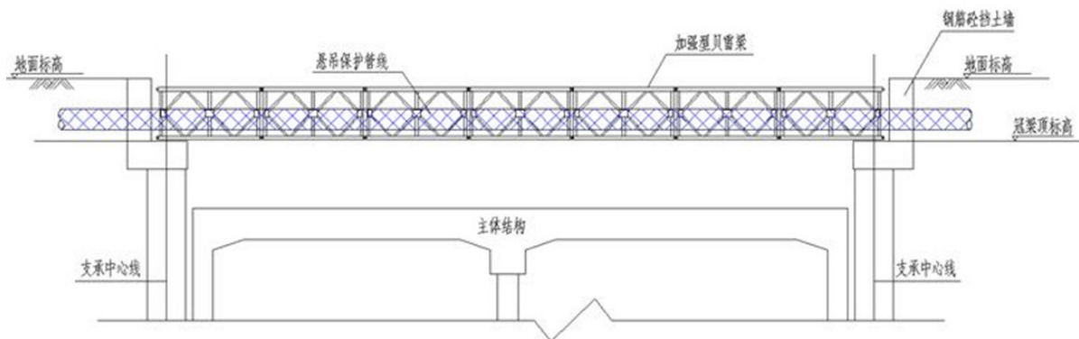
图3 管线悬吊保护示意图
