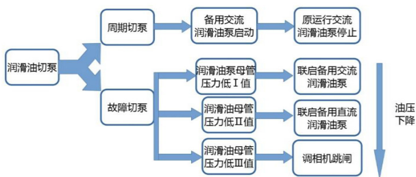
图1 润滑油系统切泵流程图
