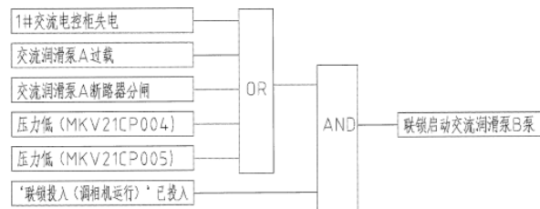
图2 联锁启动交流润滑油泵逻辑
