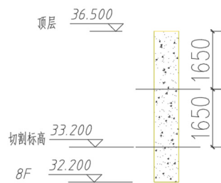
图 4 中间柱切割分块示意
