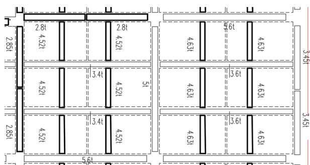
图 2 次梁 + 楼板典型分块 2
