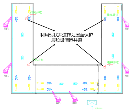
图 5 屋面层拆除示意图
