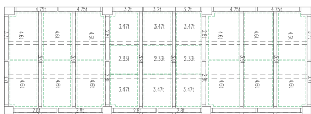
图 1 次梁 + 楼板典型分块 1
