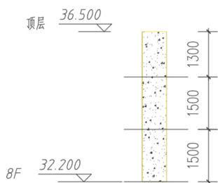
图 3 边柱切割分块示意
