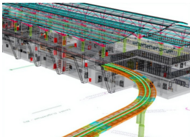
图2 BIM技术在模拟铁路施工模拟规划图
