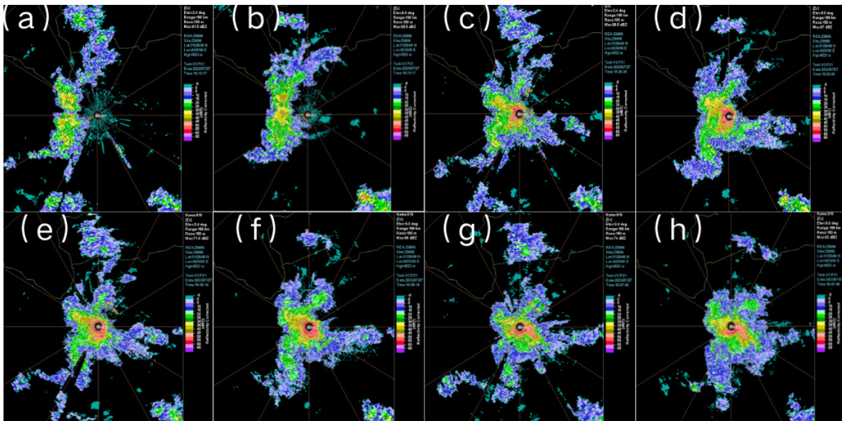
图 3 16 时 13 分 2.4^{\circ} (a)、 6^{\circ} (b) 反射率因子图, 16 时 30 分 2.4^{\circ} (c)、 6^{\circ} (d) 反射率因子图, 16 时 36 分 2.4^{\circ} (e)、 6^{\circ} (f) 反射率因子图, 16 时 47 分 2.4^{\circ} (g)、 6^{\circ} (h) 反射率因子图
