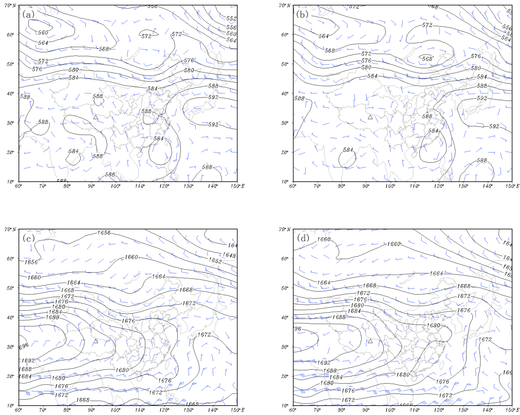
图 2 06 时 (a)、12 时 (b) 500hpa 高度场, 06 时 (c)、12 时 (d) 100hpa 高度场
