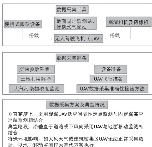
图 1 无人机空气质量监测的空间采样方案图
