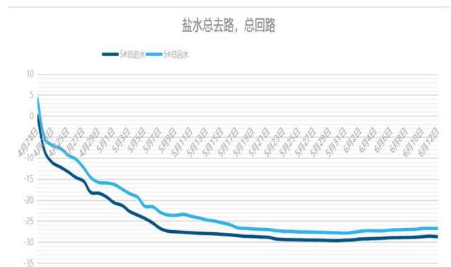
图 2 积极冷冻结盐水总去路、总回路
