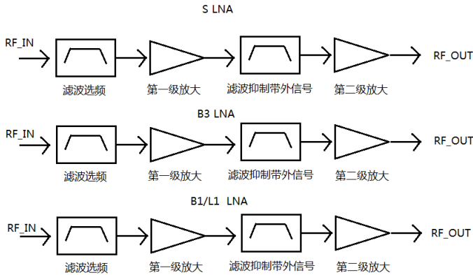
图 2 接收低噪放 LNA 设计原理框图
