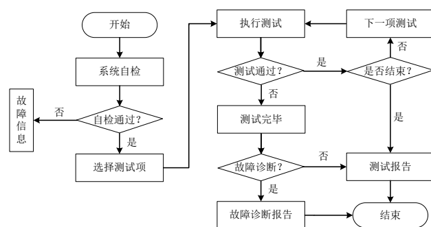
图2 软件工作流程框图
