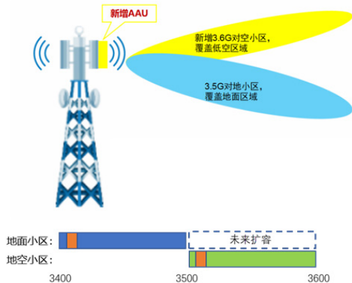
图 4 新建 3.5G 的地空载波站点示意图
