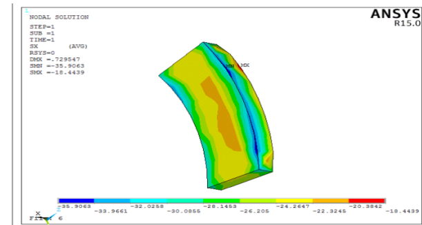
图 3 应力云图
