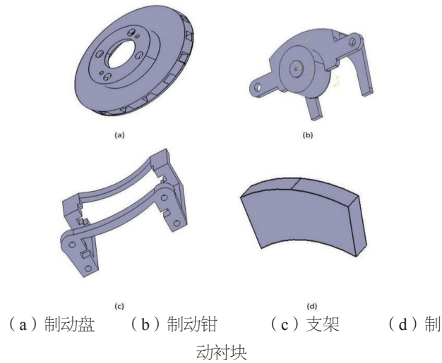
图 1 三维模型
