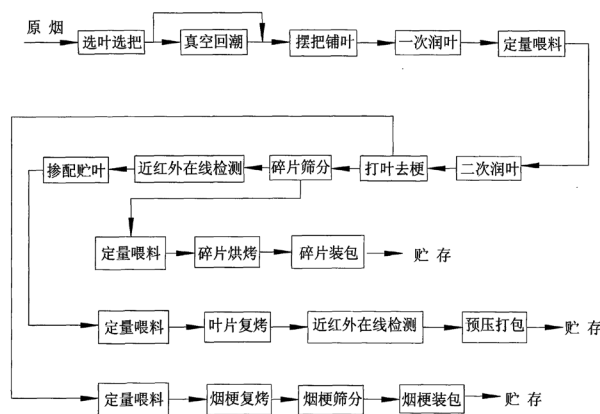
图1 均值化生产控制型打叶复烤的流程图
